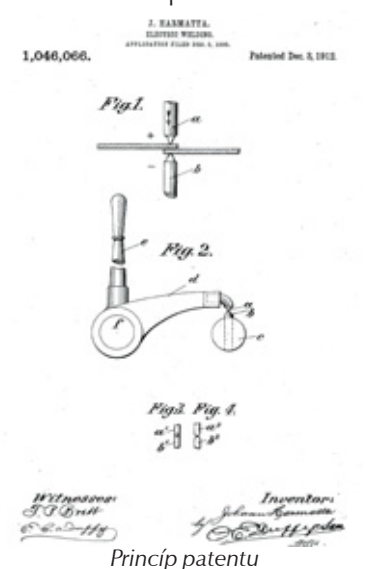
Princíp patentu
